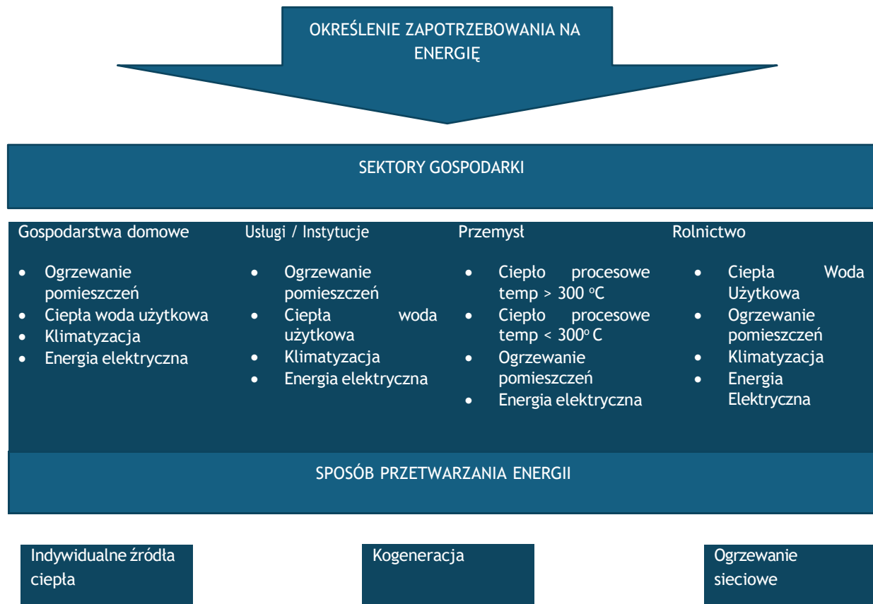
Wykres 2 Schemat bilansowania energii
